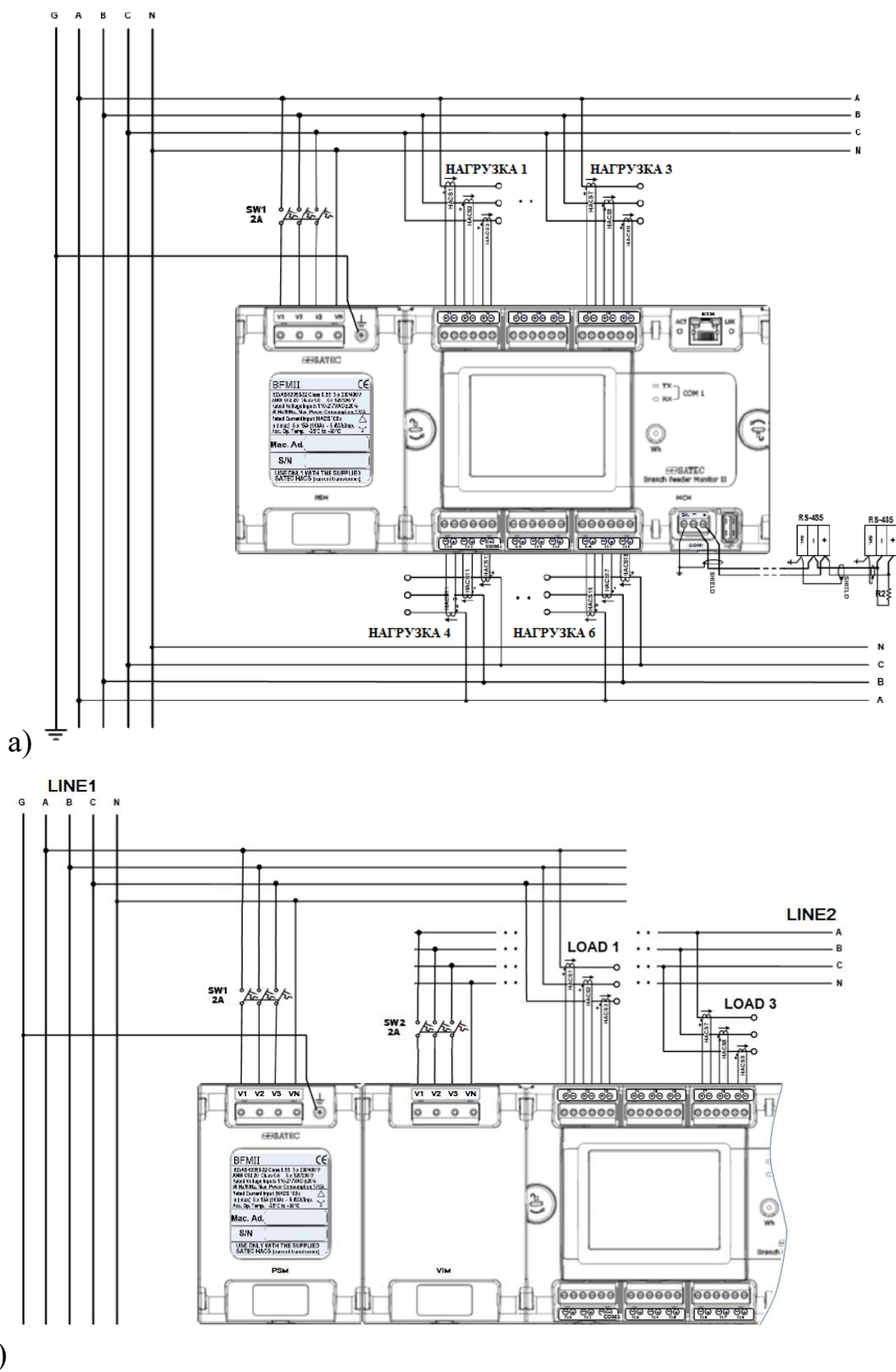
Рисунок 18 – Соединение 4LN3: а – стандарт, б – с использованием модуля VIM
