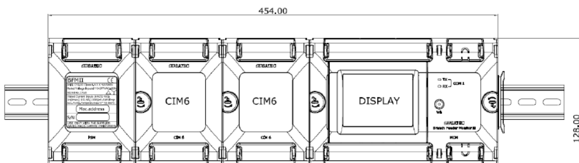
Рисунок 13 – Размеры 30-канального счётчика
