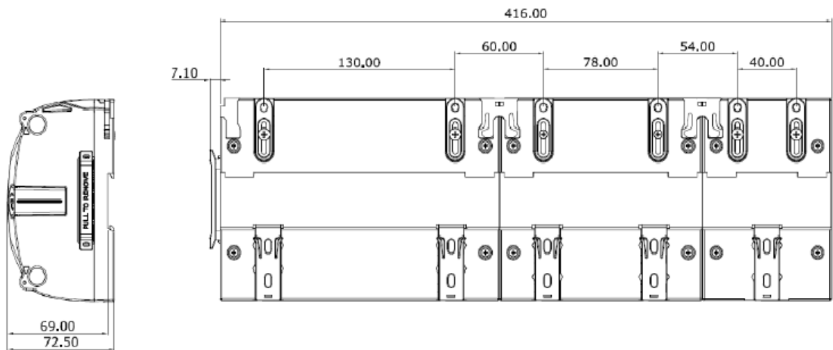
Рисунок 17 – Размеры 36-канального счётчика
