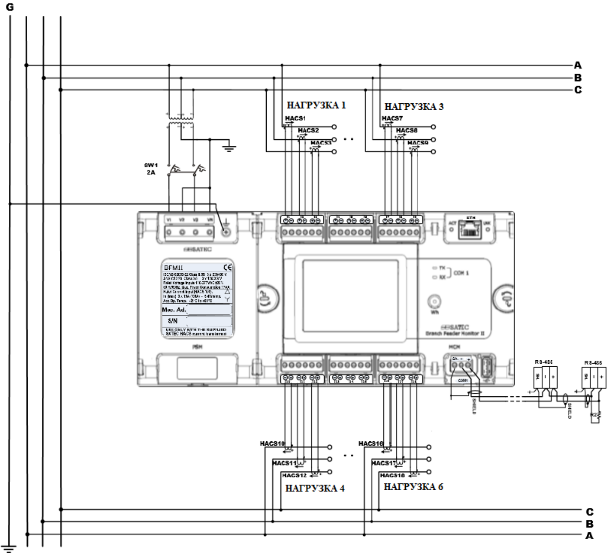
Рисунок 21 – Соединение 3Ф3
